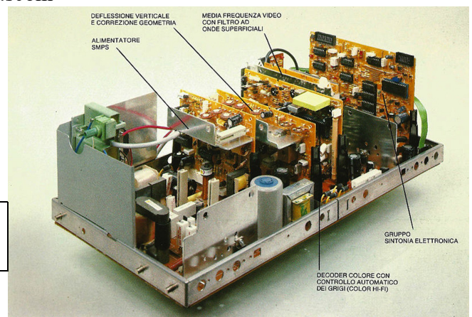
Chassis Autovox de téléviseur en couleurs
