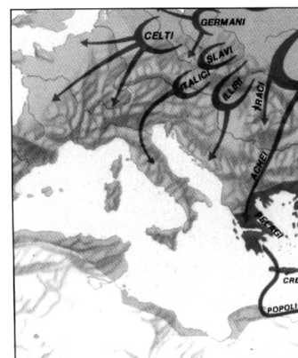
Le prime invasioni degli Italici nel Mezzogiorno, agli albori del III millennio a.C.
