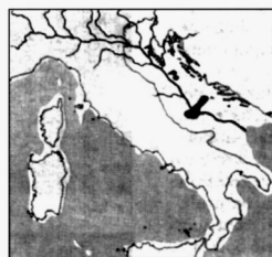
6. Il bacino adriatico, privo d'acqua, nell'Italia olocenica (12.000 anni fa) si presenta come una grande vallata
